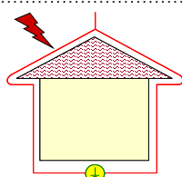
Κατασκευή με εξωτερικό ΣΑΠ – Στάθμη III & IV
