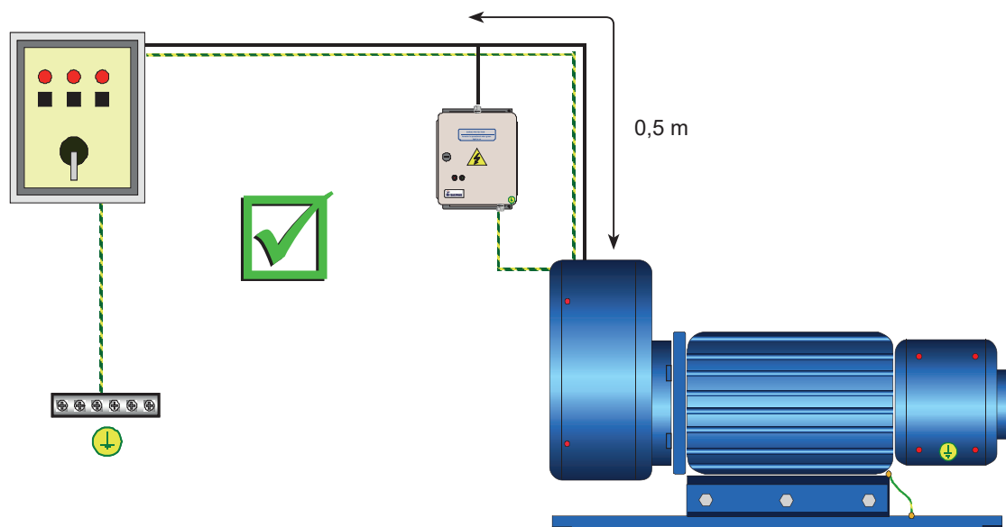
Απόσταση μεταξύ απαγωγού και υπό προστασία συσκευής < 10m (0,5m ιδανικό) – ΣΩΣΤΟ
