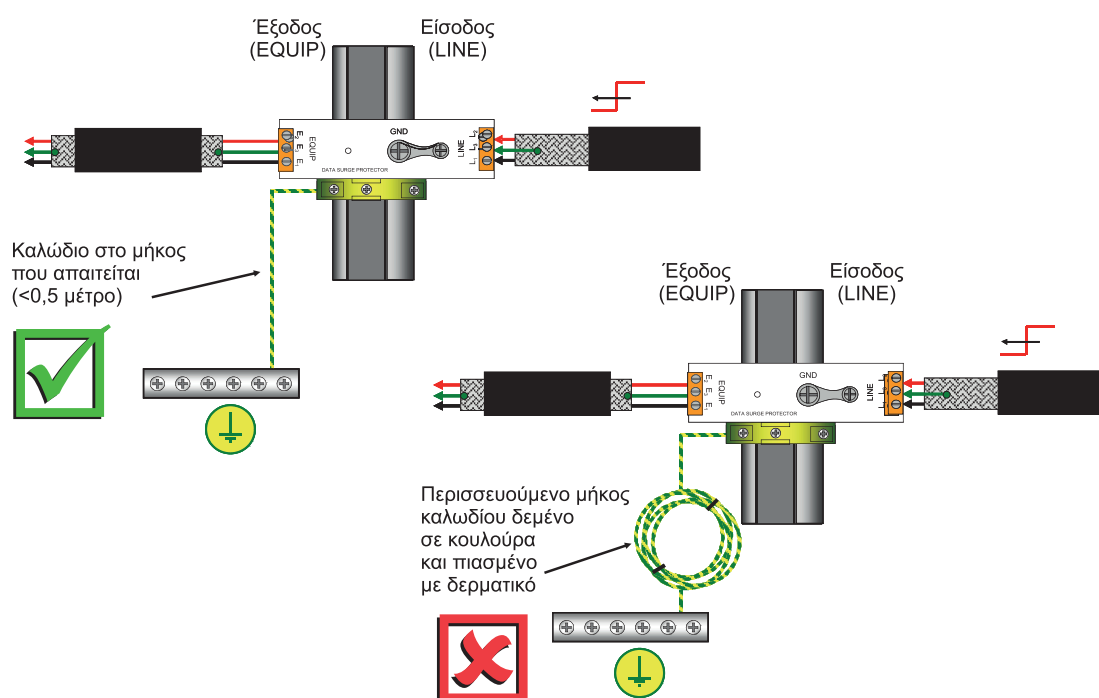
Εγκατάσταση απαγωγών κρουστικών υπερτάσεων DATA
