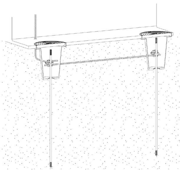
Τυπική εφαρμογή του αγωγού
