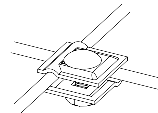
Λεπτομέρεια Β
