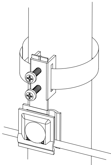
Λεπτομέρεια Α
